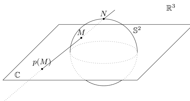
Figure 1 : Projection stéréographique.
